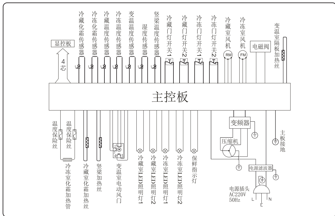
电路图 (BCD-406WMGBIW)
